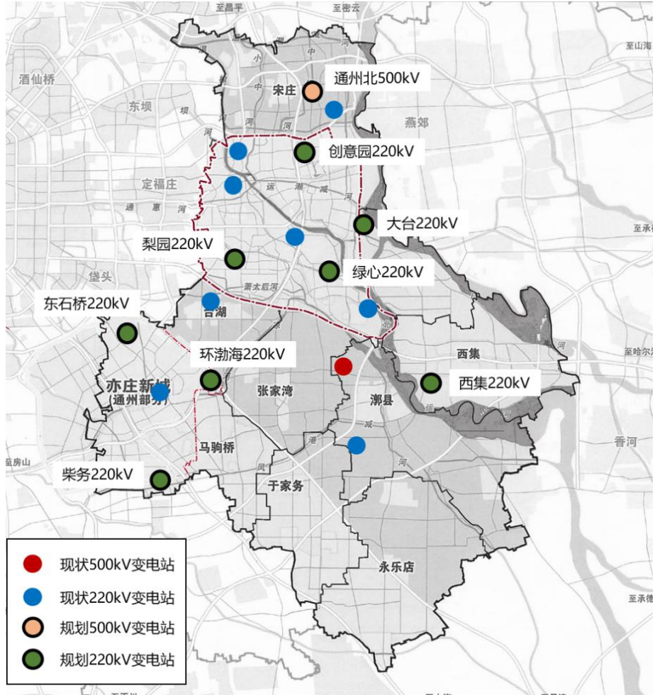
图 2-1 220 千伏及以上变电站设施布局示意图
