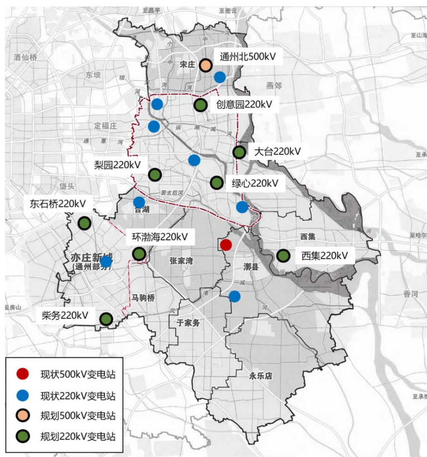
图 2-1 220 千伏及以上变电站设施布局示意图
